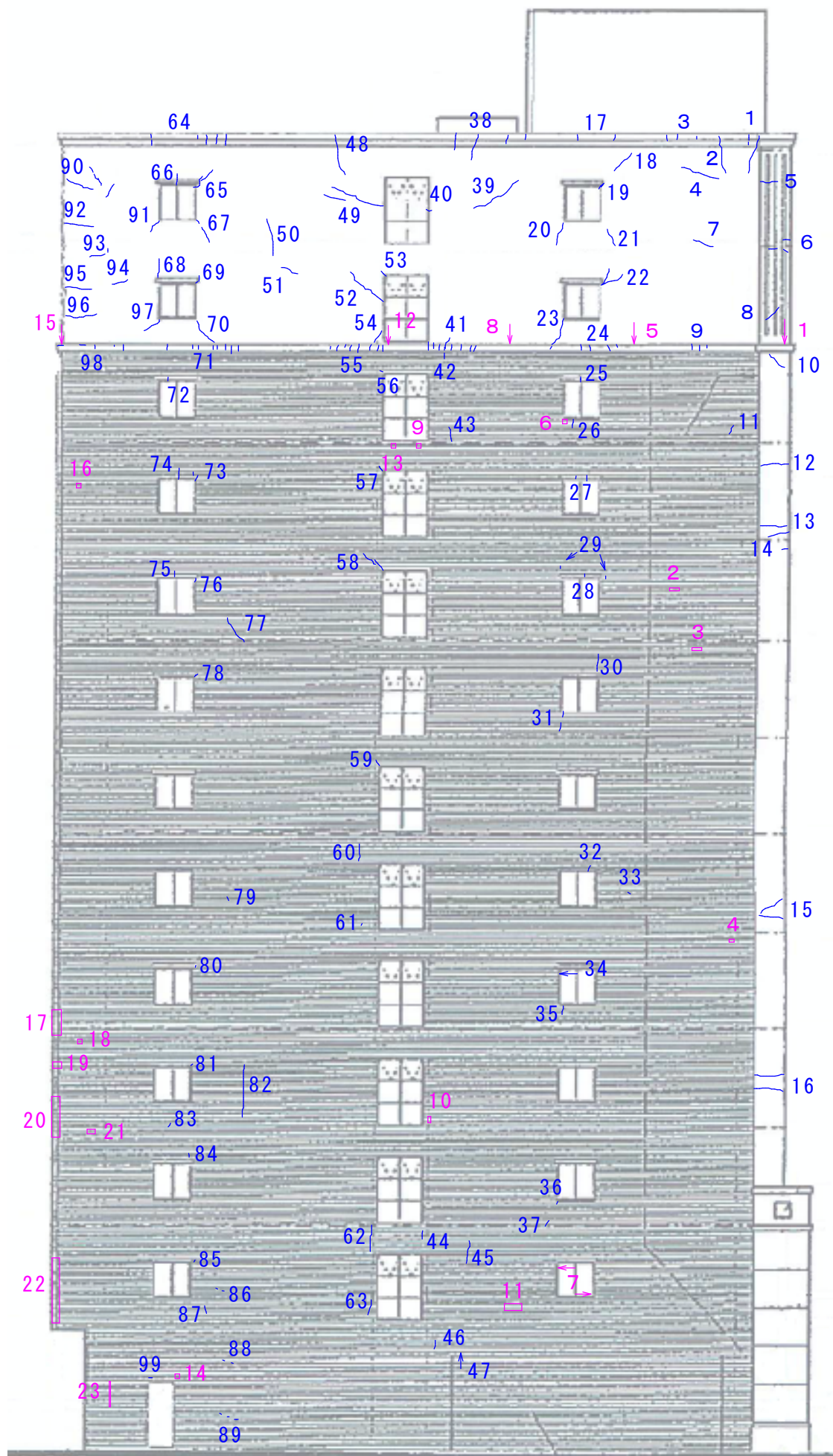
南立面図
